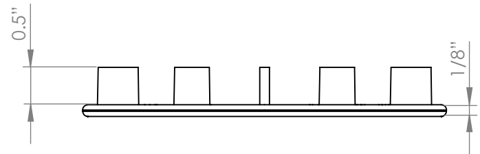
TOP SIDE
