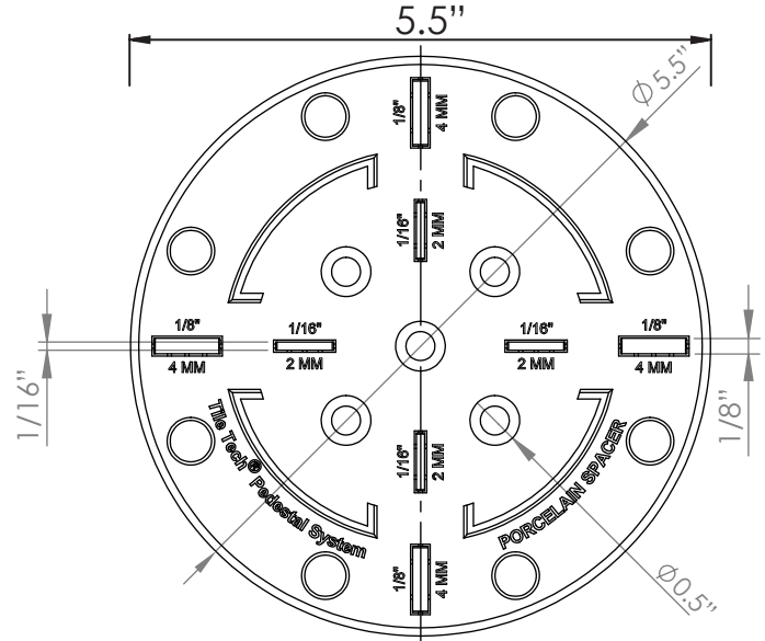
TOP SIDE
